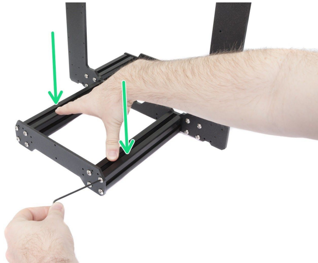
Obr. 45 - Správný způsob utažení rámu, desek a hliníkových extruzí dohromady
