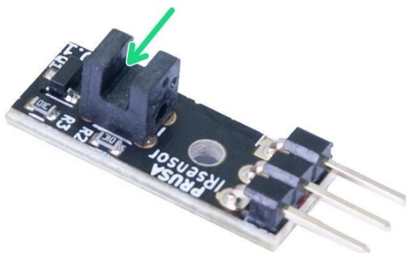
Obr. 39 - IR filament senzor
