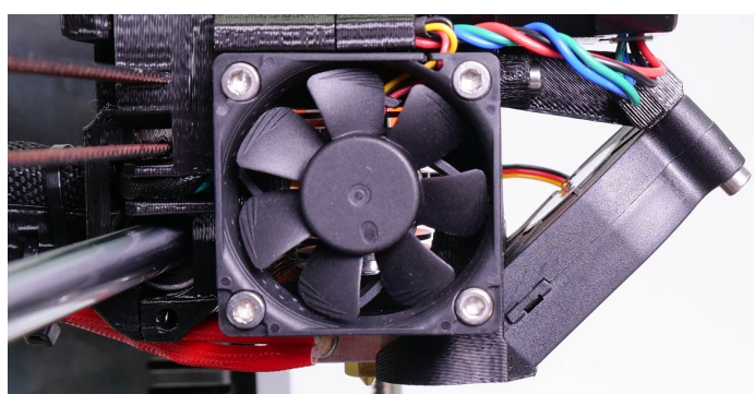
Obr. 36 - Chladicí větráček trysky značky Noctua
