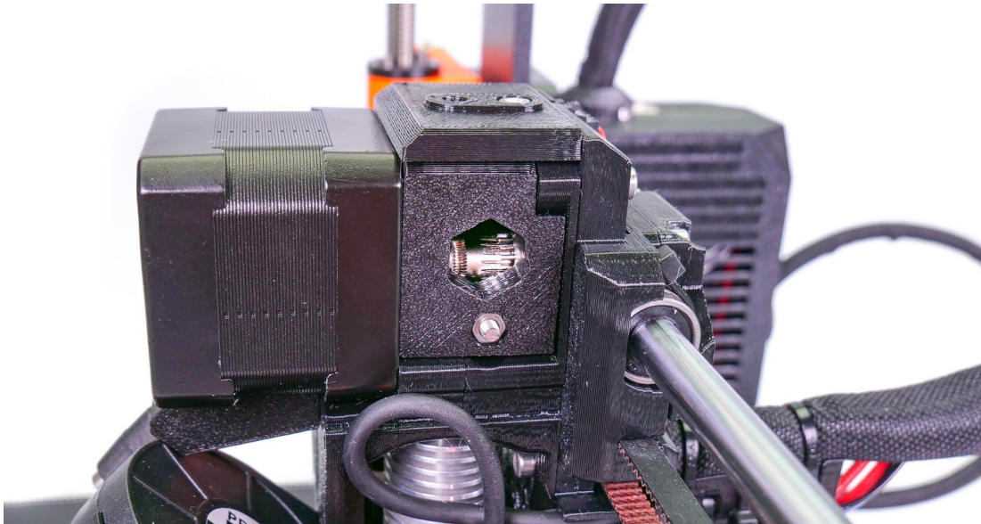
Obr. 40 - Čištění extruderu - skrz servisní otvor vidíte podávací kolečko
