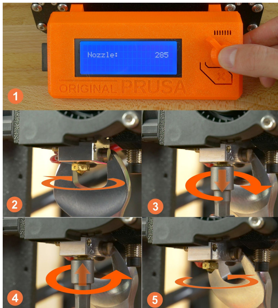
Obr. 42 - Výměna trysky
