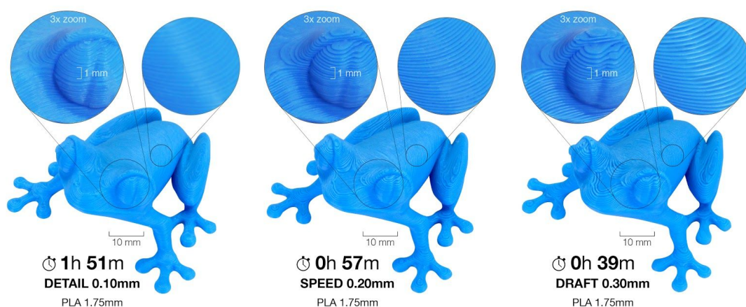
Obr. 19 - Kvalita tisku vs doba tisku
