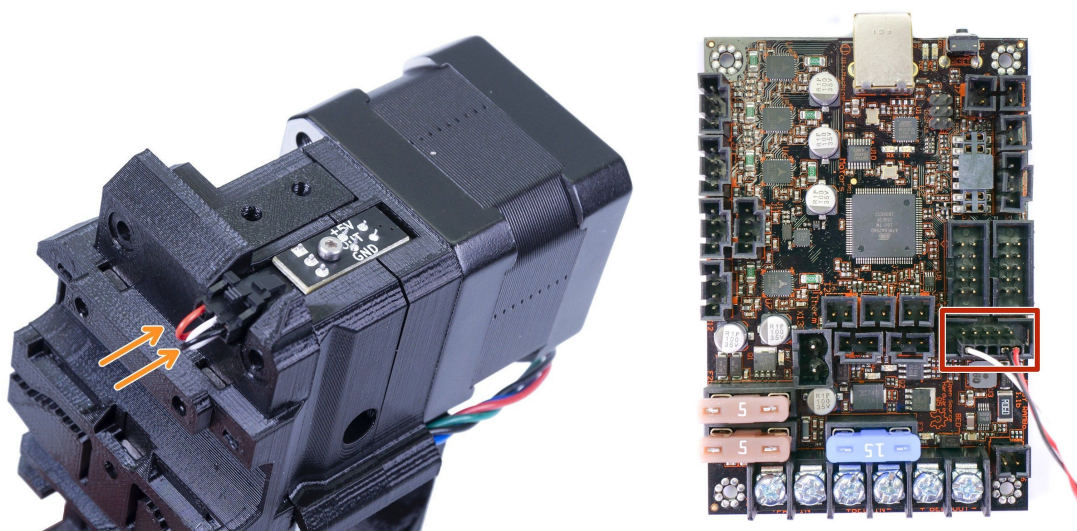
Obr. 38 - Správné usazení a připojení senzoru filamentu
