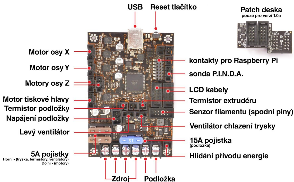
Obr. 46 - Správné zapojení konektorů
