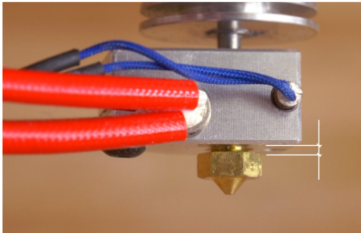
Obr. 41 – Mezera mezi tryskou a topným blokem při plném dotažení
