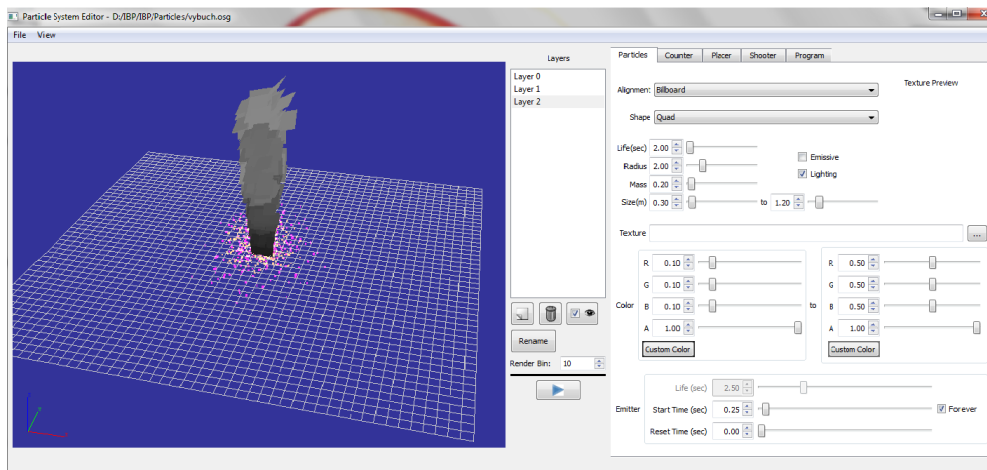
Obrázek 4.1: Particle Editor
