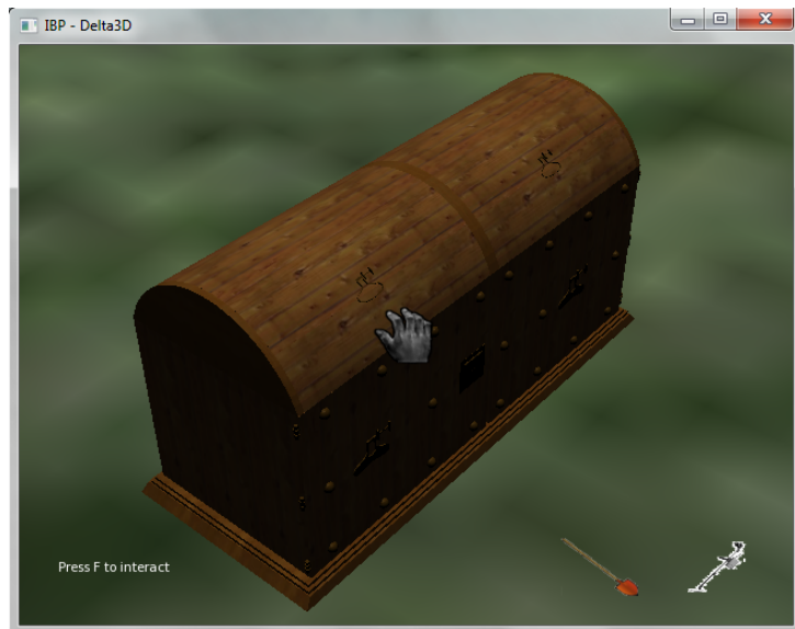
Obrázek 4.4: treasureActor
